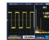
Осциллограф 10 МГц
