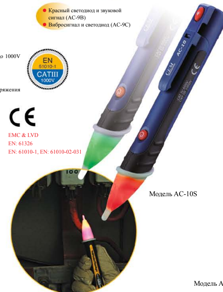
Модель AC-10
